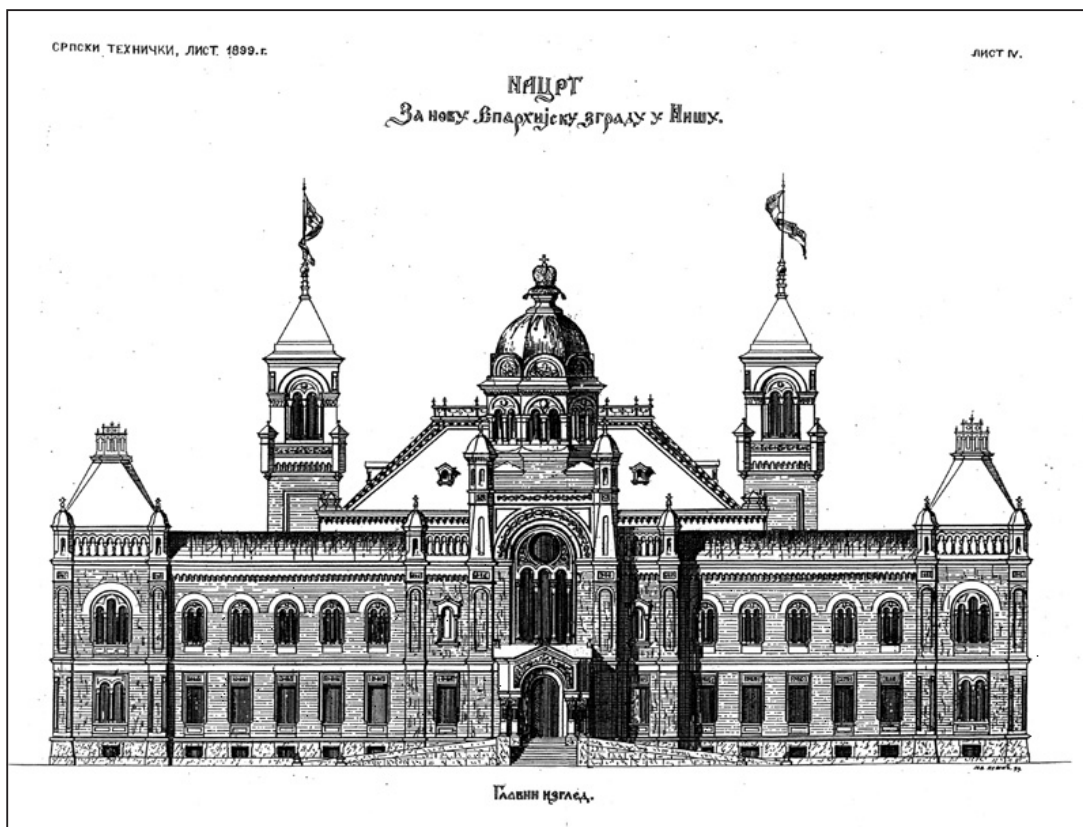
Сл. 3. Ј. Илкић, Епархијски дом у Нишу (1899), главна фасада
