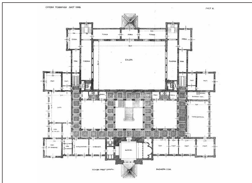
Сл. 6. Ј. Илкић, Епархијски дом у Нишу (1899), основа приземља
