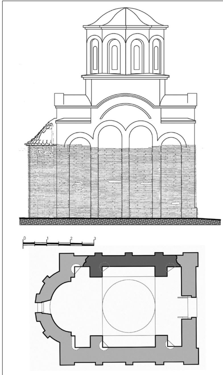
Сл. 12 Црква Св. Јована у Орљану, идеална реконструкција и основа (према арх. Јелена Ракоџија)
