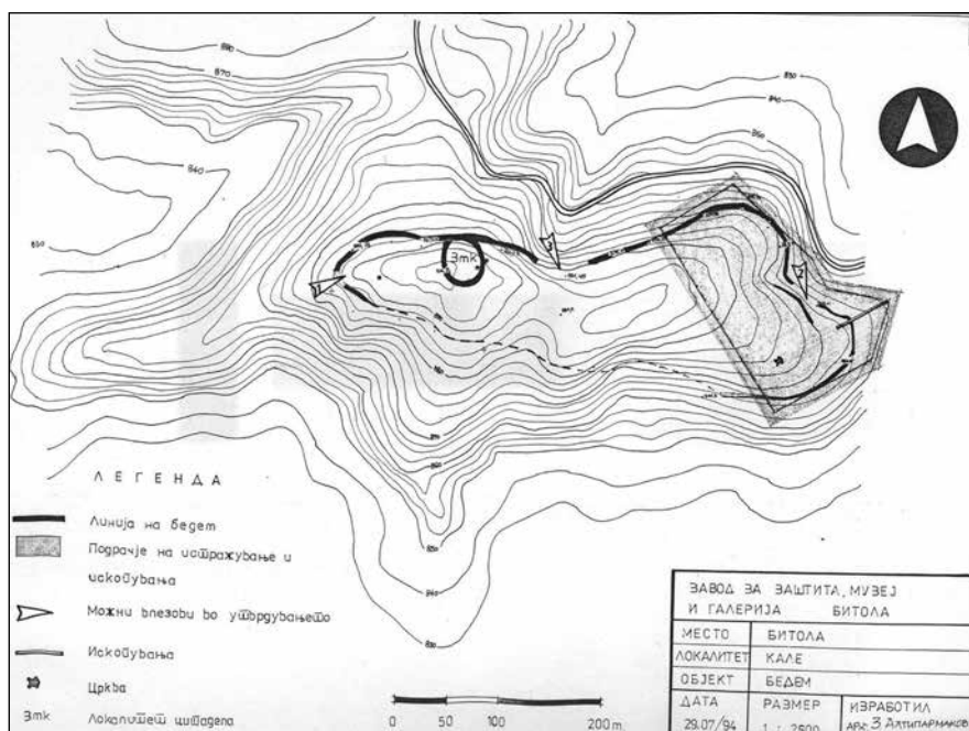
sl. 2. Мапа археолошког локалитета 'Kale bajir', 1994. (Z. Altiparmakov)
