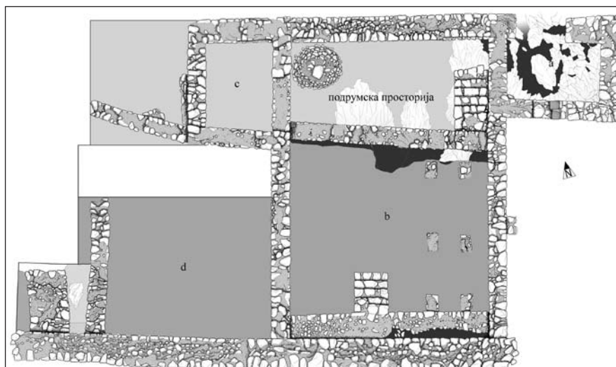
Сл. 6. Градина на Јелици. Објект VI, основа.
