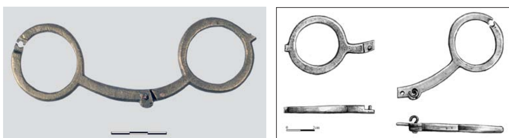
Сл. 10а-б. Градина на Јелици, Објект VI. Полијелеј III. Abb. 10а-б. Die Gradina auf der Jelica, Objekt VI. Polykandelon III.
